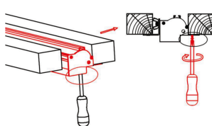
5. Parafuse o perfil em uma estrutura para suporte (madeira)
