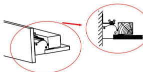
6. Intale o forro de drywall e parafuse o perfil em uma estrutura para suporte (madeira)
