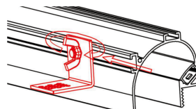
3. Fixe a presilha no perfil
