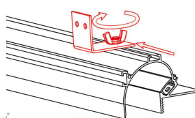
3. Fixe a presilha no perfil
