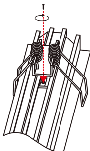
4. Aperte os parafusos da mola
