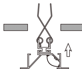
6. Após fazer o recorte no teto, insira o perfil pressionando a mola para passar pelo recorte
