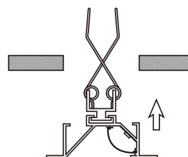
6. Após fazer o recorte no teto, insira o perfil pressionando a mola para passar pelo recorte
